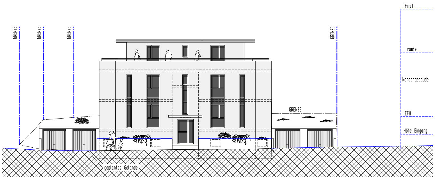
ANSICHT NORD
