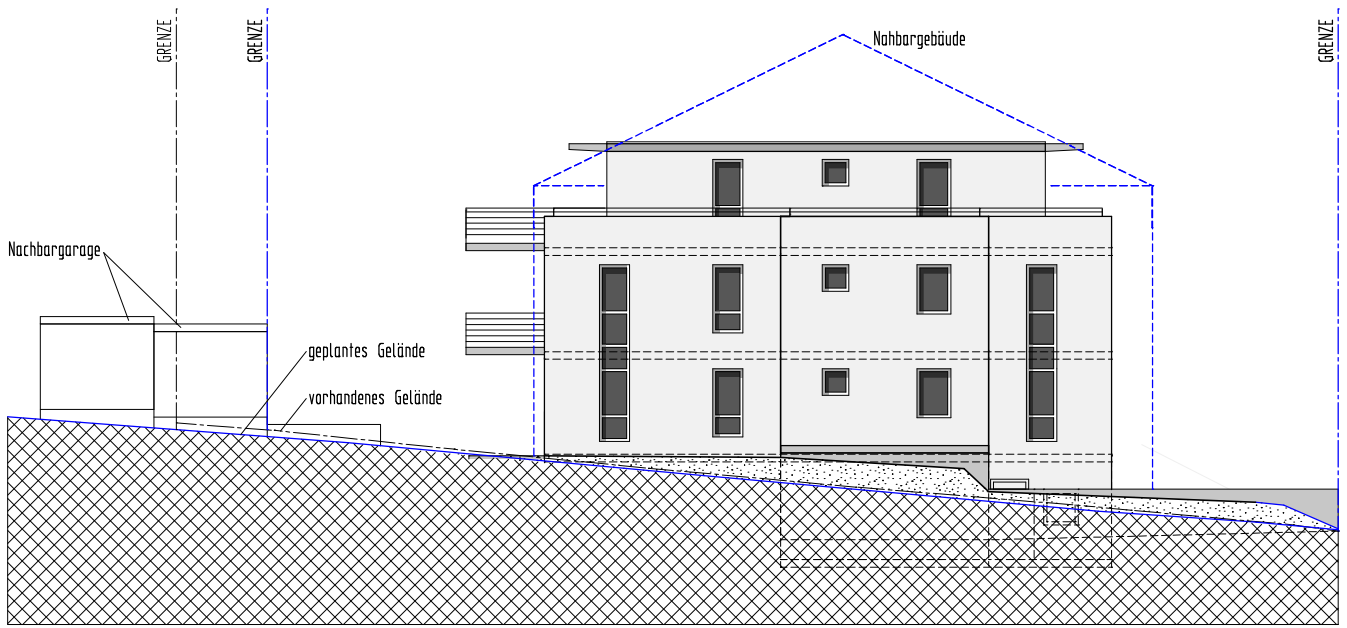
ANSICHT OST
